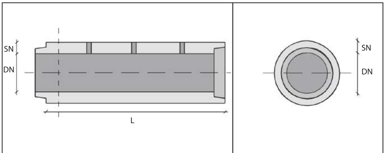
SEZ. LONGITUDINALE
