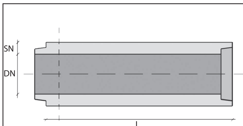
SEZ. LONGITUDINALE
