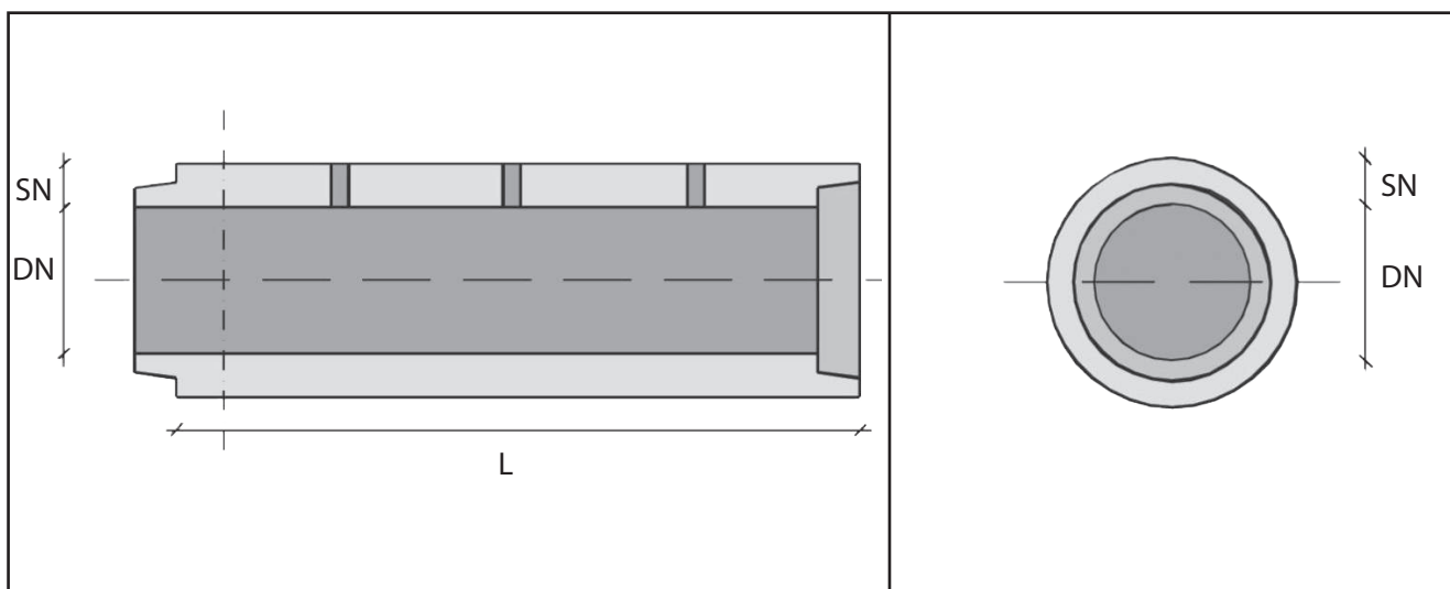
SEZ. LONGITUDINALE
